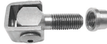
Torband Edelstahl · Inox mit Schweißmutter M20 Art. 9.04.5000 M24 Art. 9.04.5030
