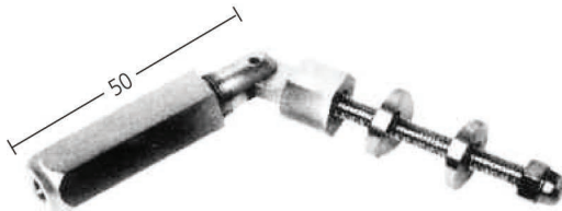
Seilspanner , 6-teilig, für Rohr 42,4 mm, Seil 4 mm Rope winder , 6 parts, for tube 42,4 mm, rope 4 mm Art. 9.07.0200
