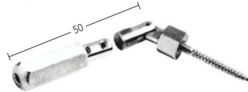
Seilspanner , 4-teilig, für Flachanschluss, Seil 4 mm Rope winder , 4 parts, for flatmount, rope 4 mm Art. 9.07.0210
